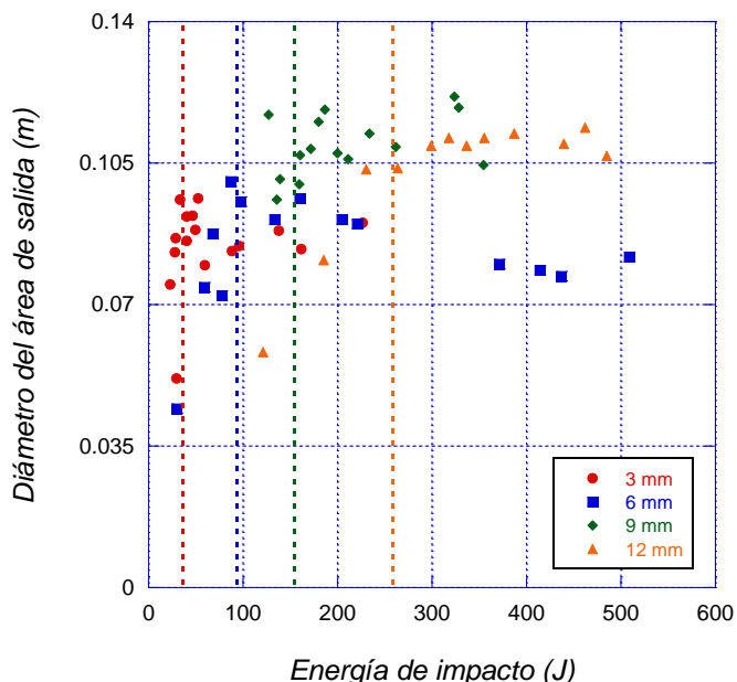
Figura 8. Evaluación del daño en la superficie de salida del laminado en función de la energía de impacto para laminados de fibra de vidrio E en resina poliéster
