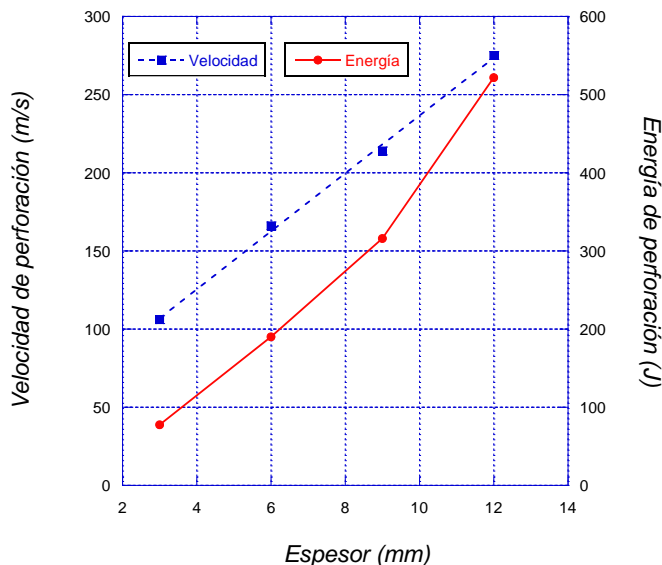
Figura 3. Energía y velocidad mínima de perforación en función del espesor del laminado de fibra de vidrio E en resina poliéster
