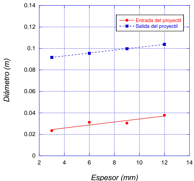
Figura 9. Diámetro del daño para la energía mínima de perforación en función del espesor de los laminados de fibra de vidrio E en resina poliéster
