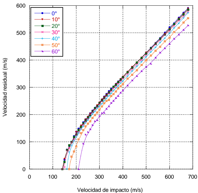
Figura 8. Velocidad residual vs. velocidad de impacto en función del ángulo de oblicuidad del proyectil para las placas espaciadas.
